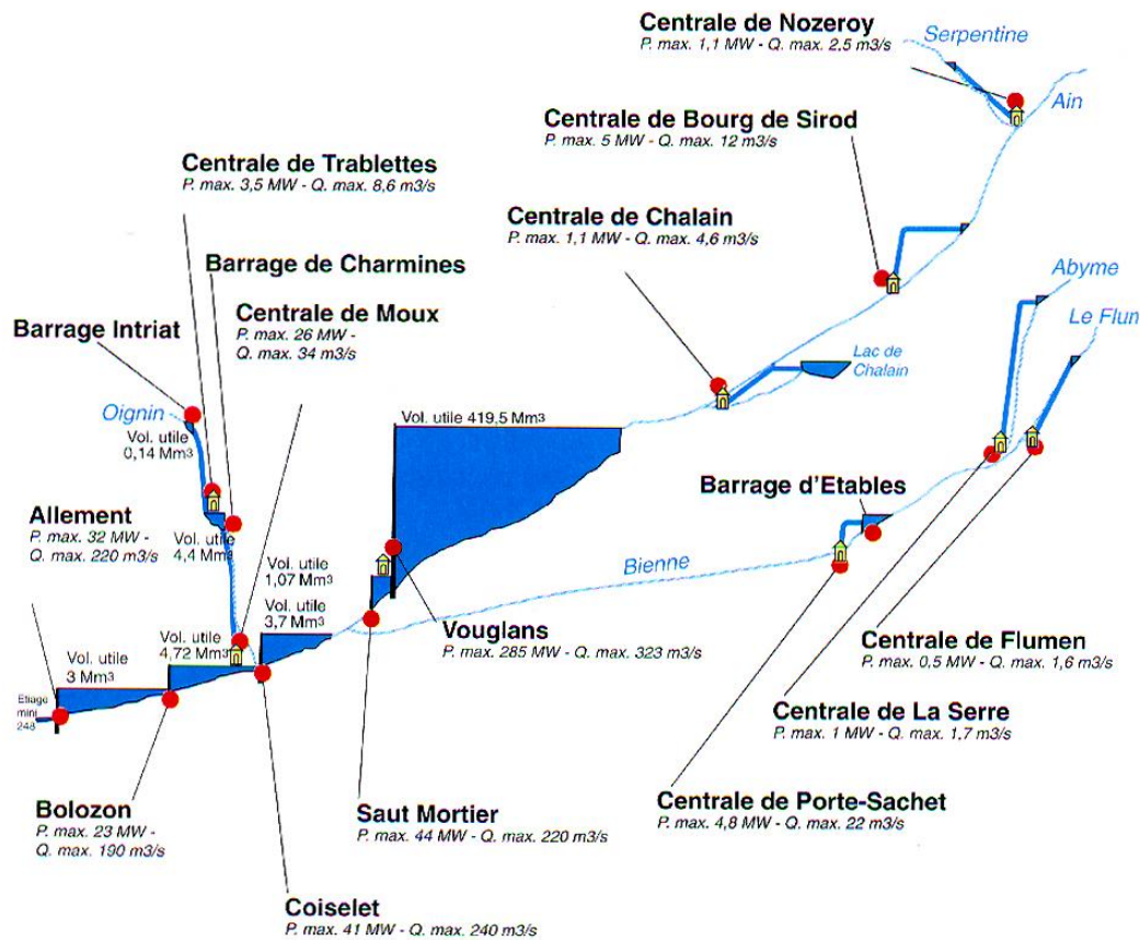
Figure 2.28 : Schéma récapitulatif de l'ensemble des barrages hydroélectriques et microcentrales exploités par EDF sur l'amont du bassin versant de la rivière d'Ain (Source EDF)
