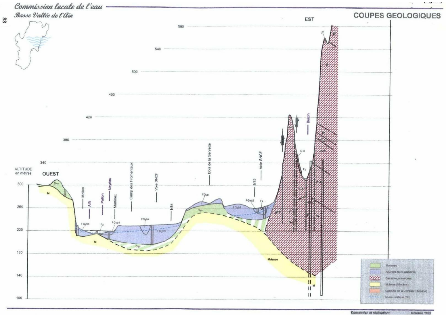
Figure 2.4 : Coupe géologique de Rignieux-le-franc à Vaux-en-Bugey (Horizons, 1999)
